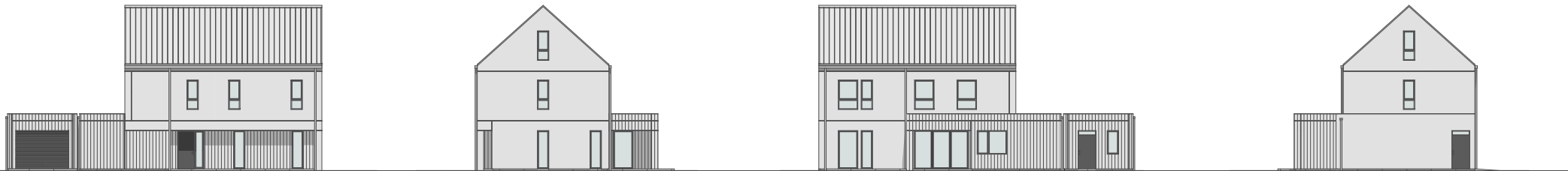
ELEWACJA FRONTOWA
